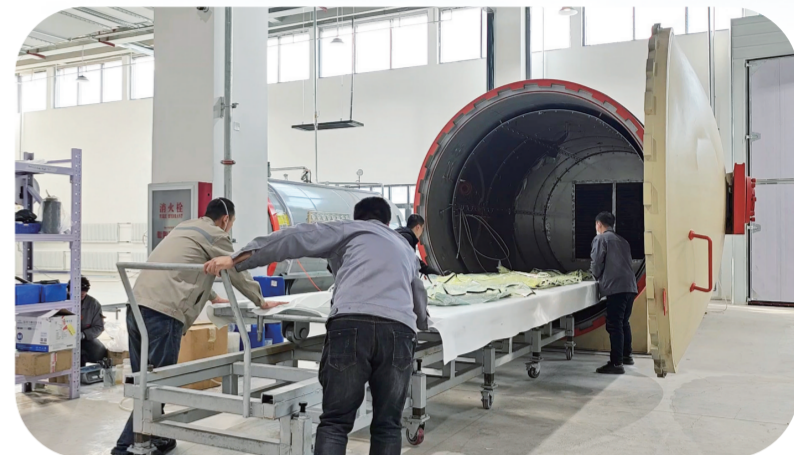
操作人员正在进行机身复材成型生产。
