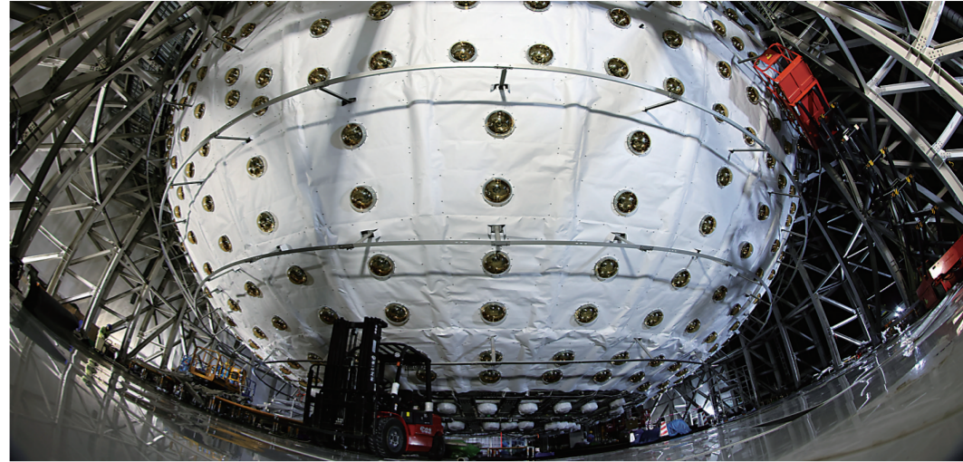
11月22日拍摄的探测器。我国大科学装置——江门中微子实验的探测器主体日前建成。江门中微子实验位于广东江门开平市，将以测量中微子质量顺序为首要科学目标，同时开展多项重大前沿交叉研究。记者日前探访探测器主体建成后的江门中微子实验。 新华社记者 金立旺 摄
