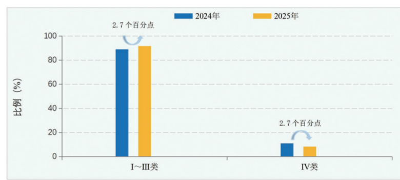
全省109个国控断面水质类别比例年际比较图。
