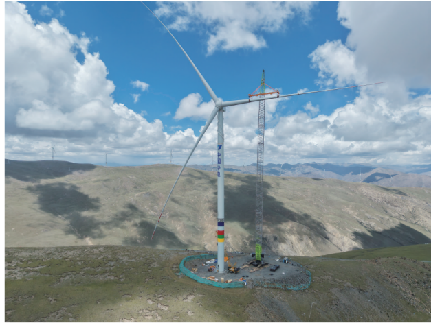
首台风机整体吊装完成(6月18日摄)。6月18日，中建二局承建的西藏华电珠球440MW风电基地一期150MW风电项目首台风机顺利在西藏山南市琼结县完成吊装，这座最高点海拔达5350米的超海拔山地风电工程迎来施工关键节点，标志着项目全面转入风机设备安装攻坚阶段。新华社发
